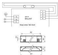
Technische Daten Philips HF-P 1 14-35 TL5 HE III 220-240V
